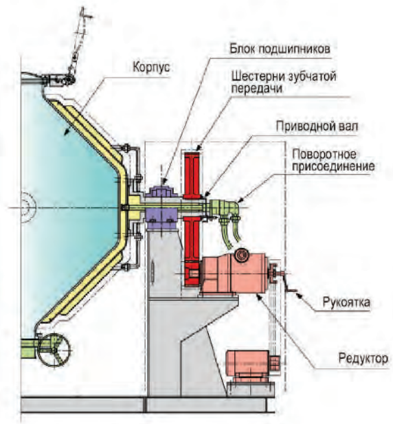
Привод с зубчатой передачей
