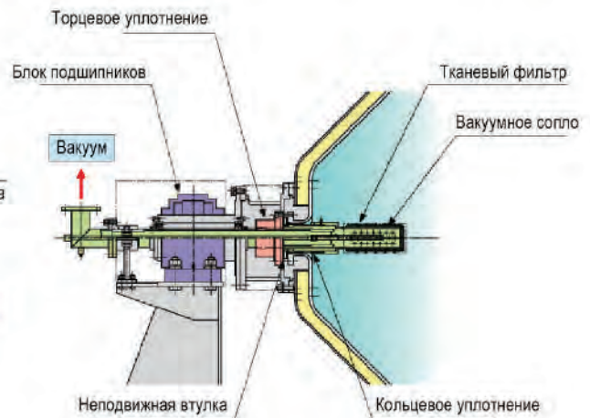
Вращающееся вакуумное сопло
