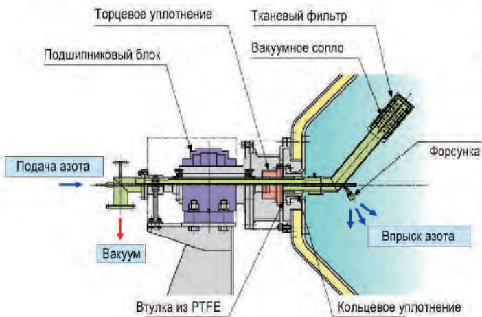
Неподвижное вакуумное сопло
